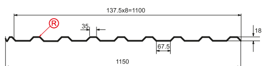
Профилированный лист МП-20x1100-В, R Толщина материала 0,4–0,8 мм
