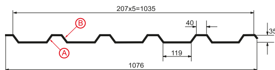
Профилированный лист МП-35x1035-В Толщина материала 0,45–0,9 мм
