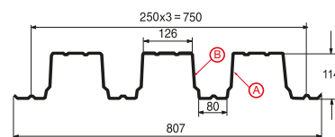
Профилированный лист Н-114x750-А, В
