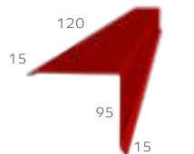
Планка торцевая 95x120x2000
