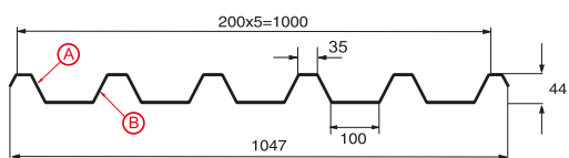
Профилированный лист С-44x1000-А Толщина материала 0,45–0,8 мм
