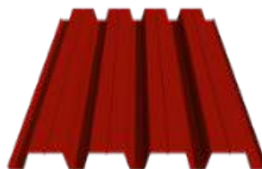
Профилированный лист МП-35x1035-В Толщина материала 0,45–0,9 мм
